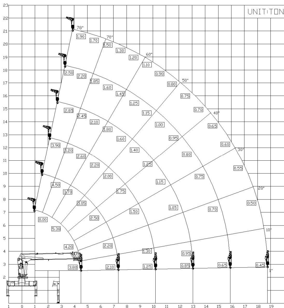
Рис. 4 График рабочей зоны, соотношение вылета, угла подъема стрелы и подъема крюковой подвески.
