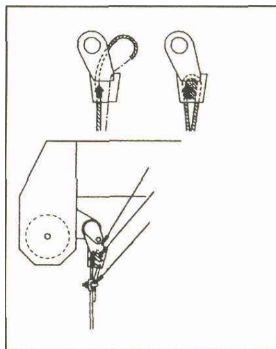
Обжимка каната
