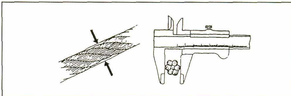
Проволока (шаг) Жила
