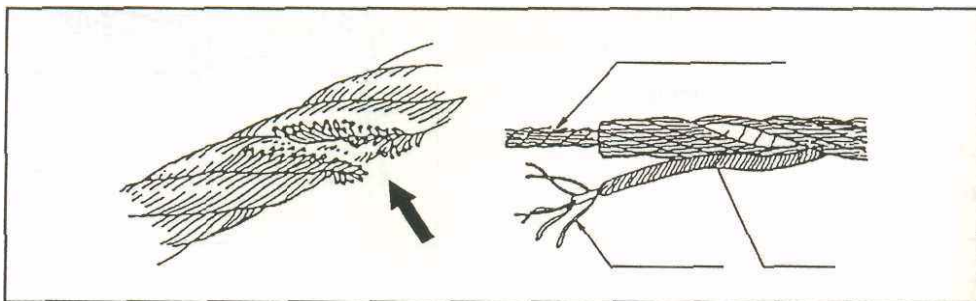
Проволока (шаг) Жила
