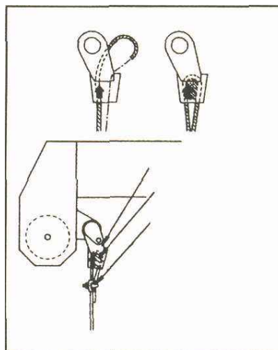
Обжимка каната
