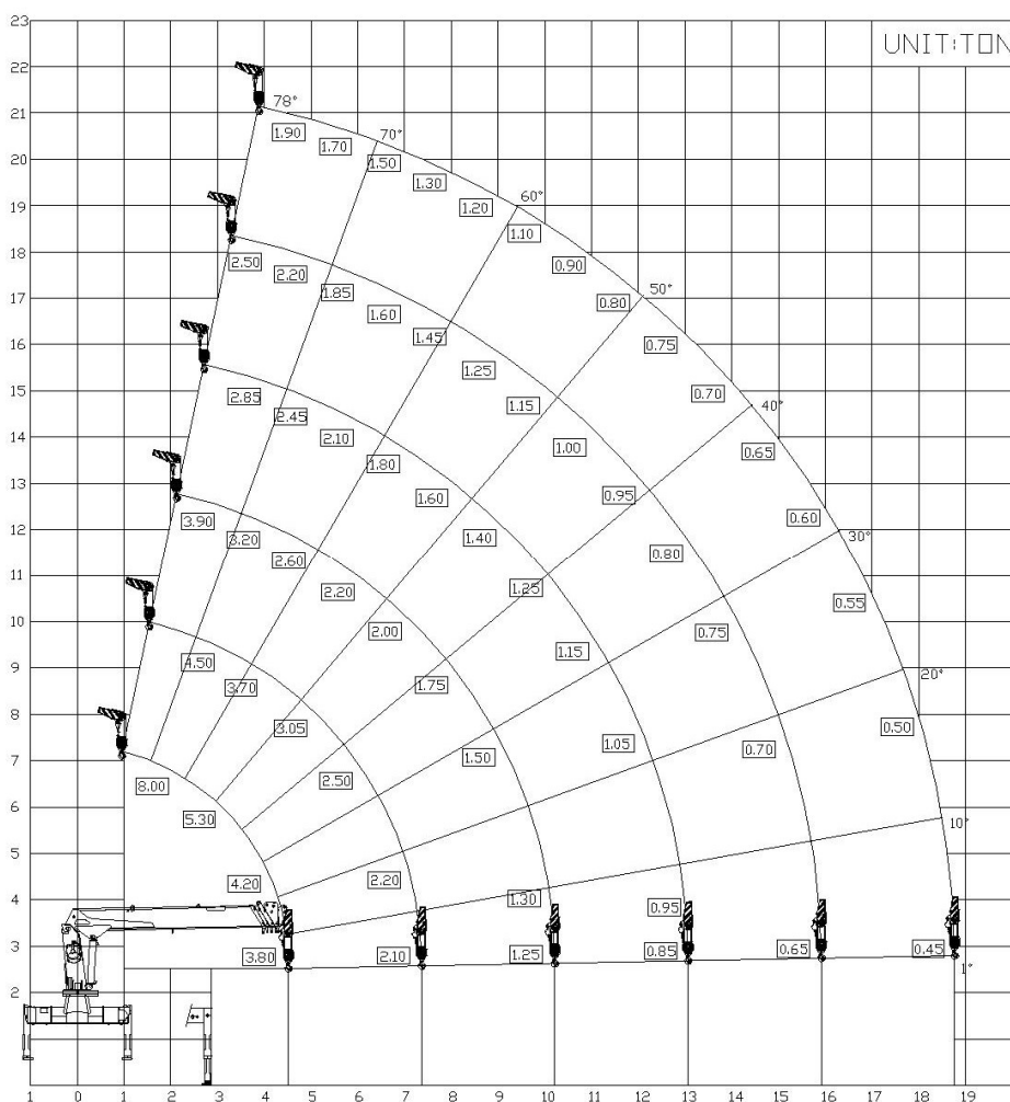
Рис. 2 Диаграмма высотных характеристик КМУ модели HGC756Plus
