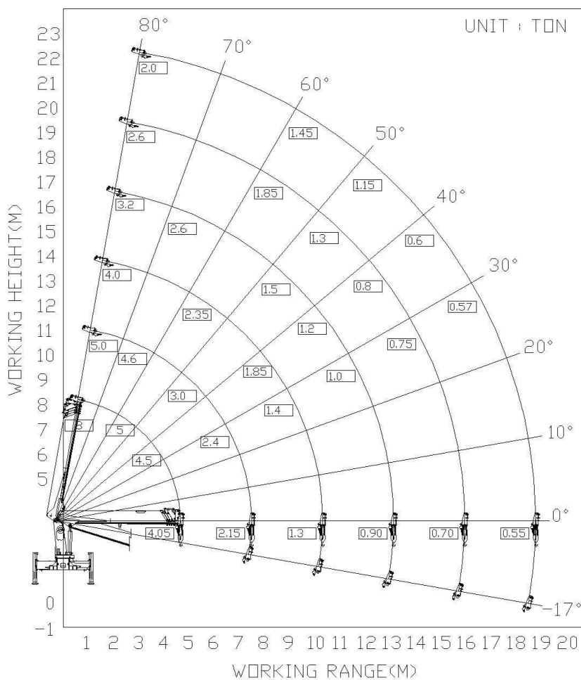
Рис. 2 Диаграмма высотных характеристик КМУ модели HGC976
