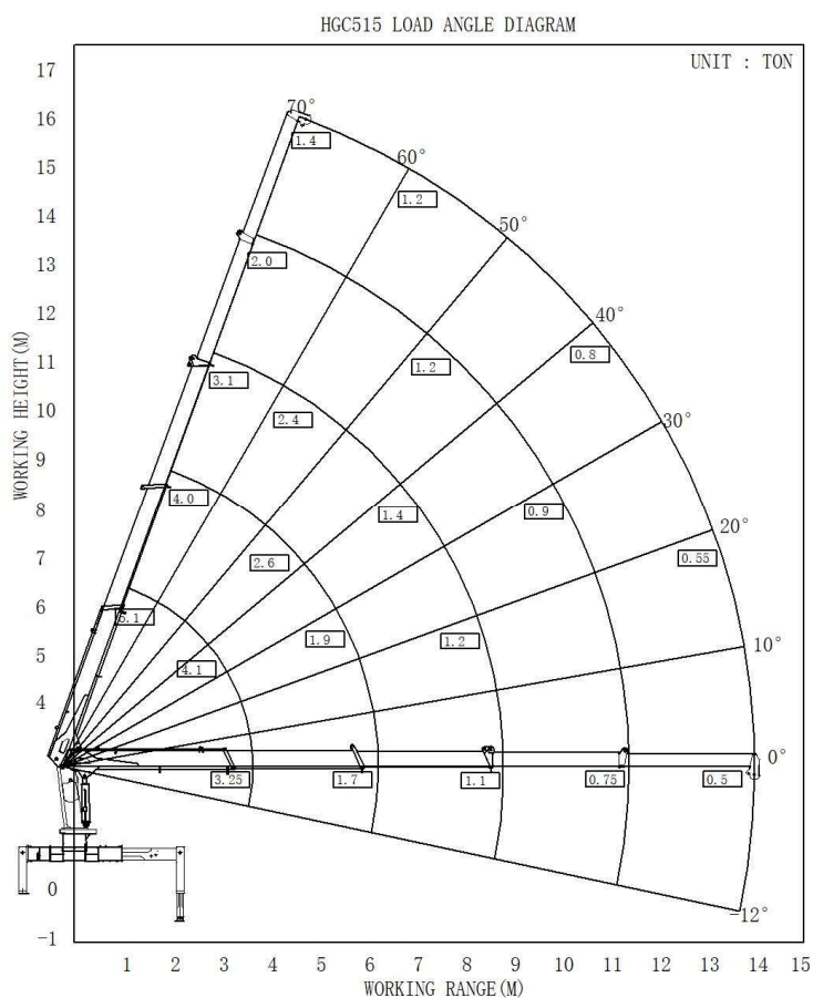
Рис. 2 Диаграмма высотных характеристик КМУ модели HGC515
