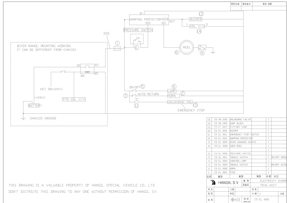
Рис. 4 КМУ модели HGC515 Схема электрическая принципиальная
