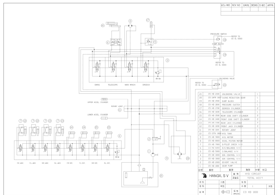
Рис. 5 КМУ модели HGC515
