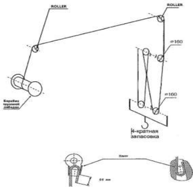
Рис. 7 Схемы запасовки грузового каната.
